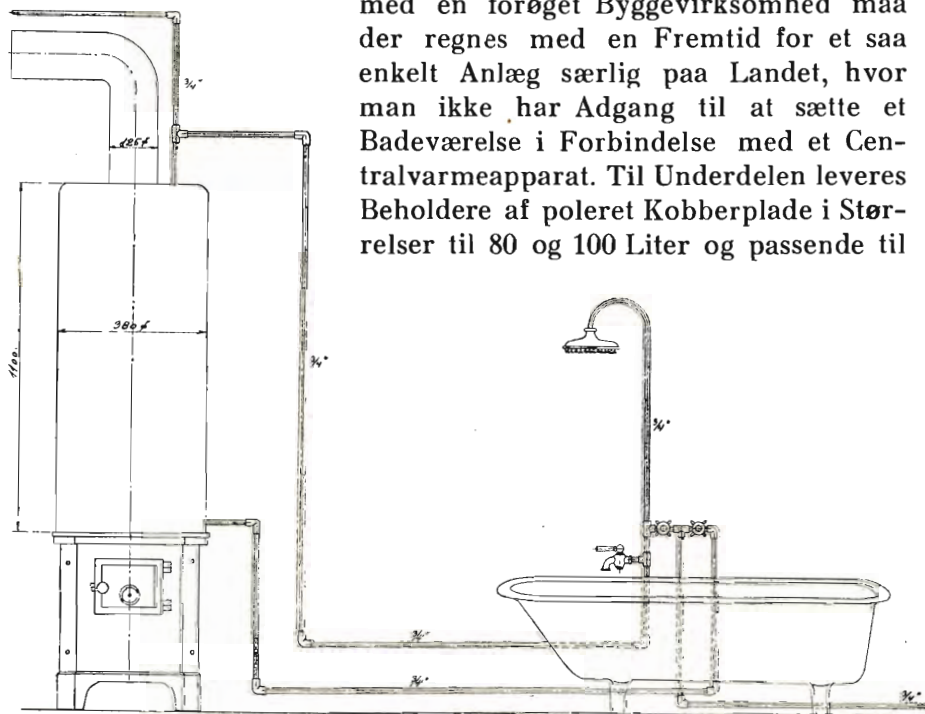
Fig. 2. Skematisk Badeovnsarrangement beregnet til Fyring med Brænde.
