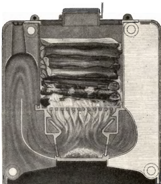
Fig. 8. De forenede Jernstøberiers Kedel Type DVI til Brændefyring, opstillet første Gang paa Astrup ved Jyderup.
