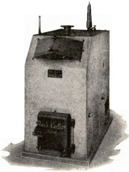
Fig. 7. Brændefyringskedel fra A/S Recks Opvarmnings Co. leveret til Graasten Slot. Højde 1800 mm, Bredde 1350 mm, Dybde 1600 mm. Hedeflade 18 m 2 . Brændelængde 0,63 m.
